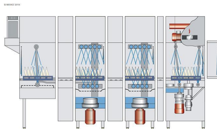
Doorsnede machine schematisch weergegeven
